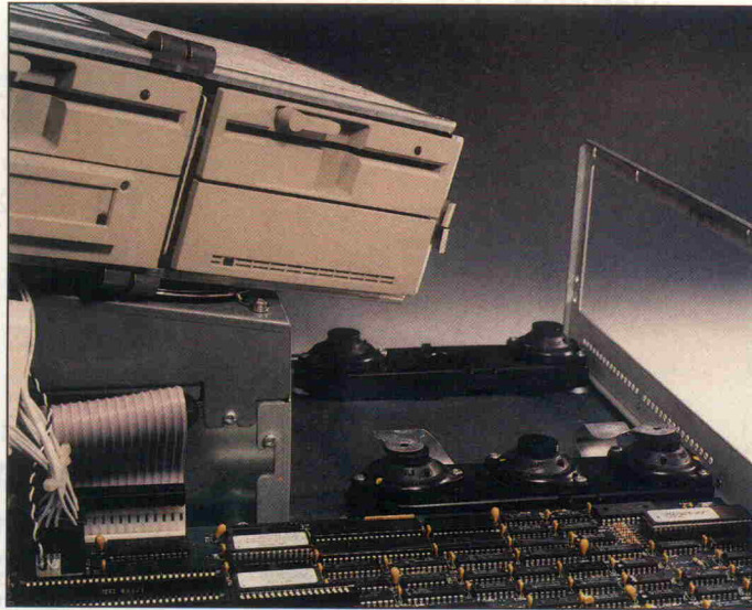
Der Blechkasten, in dem die Massenspeicher als kompakte Einheit untergebracht sind, ruht auf Stoßdämpfern. Ein professionelles Konzept.
