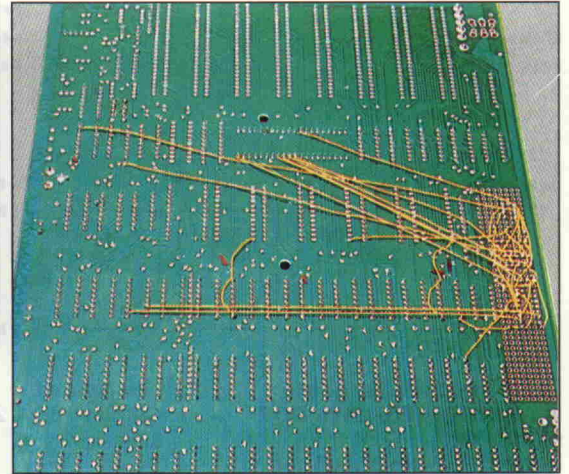
Die Zusatzlogik läßt sich bequem auf dem freien Rasterfeld der Hauptplatine unterbringen. Die Verdrahtung versteckt sich unter dem Motherboard.
