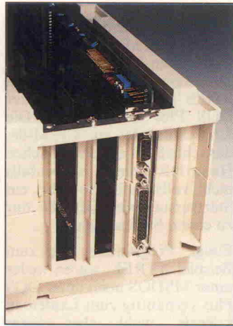
Eine EGA-Karte, wie sie hier aus dem Erweiterungspalt lugt, läßt sich leider nur sehr eingeschränkt nutzen. Ärgerlich, aber nicht so tragisch: gut ummantelte Stecker können mit den breiten Kunststoffstegen kollidieren.
