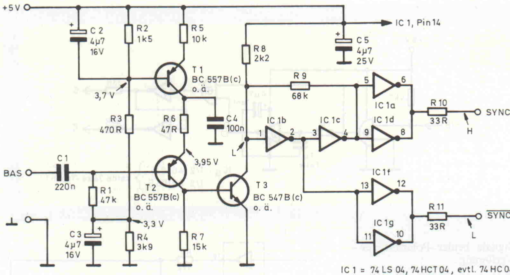
Das Schaltbild des Takt-Trenners. Weiteres – von der Funktionsbeschreibung bis zum Platinenlayout – finden Sie in c't 9/86.
