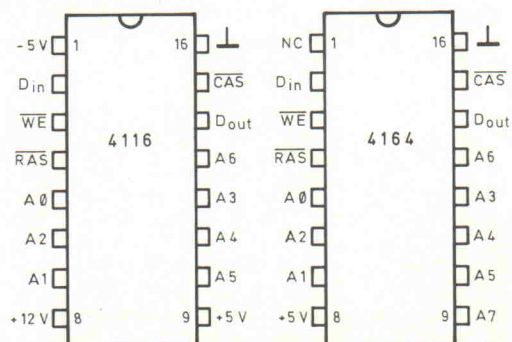
Die Pin-Belegung des 4164 ist mit der des im Apple verwendeten 4116 fast identisch.
